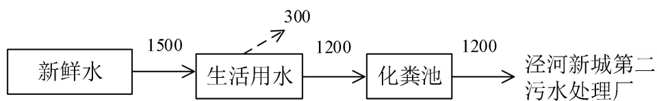
图 2-1 项目水平衡图 (单位: \text{m}^3/\text{a} )
